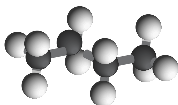
Butano - C 4 H 10
