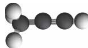
Metilacetileno - C 3 H 4
