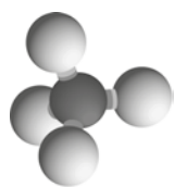
Metano (Gas Natural) - CH 4
