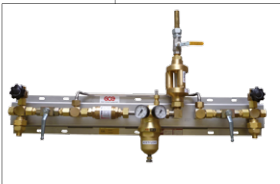
Panel de regulación y cambio manual de gran caudal de acetileno MM400 - 2 ACE
