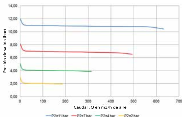
Curva de caudal del S151 con 17 bar (246Psi) de presión de entrada (P1)
