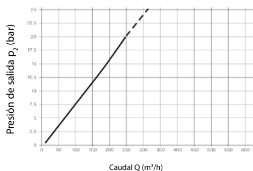
RELACIÓN ENTRE EL CAUDAL Y LA PRESIÓN DE SALIDA - VPK 251
