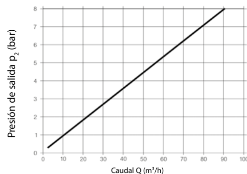
RELACIÓN ENTRE CAUDAL Y PRESIÓN DE SALIDA - VPKU 91
