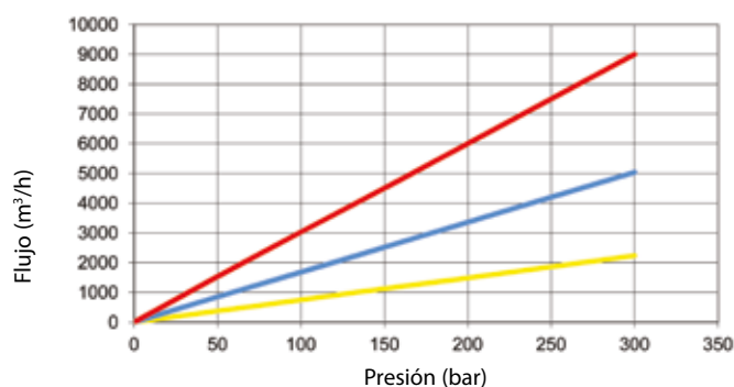
Curva de capacidad de flujo de válvulas de línea GCE
