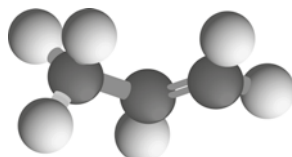
Propileno - C 3 H 6
